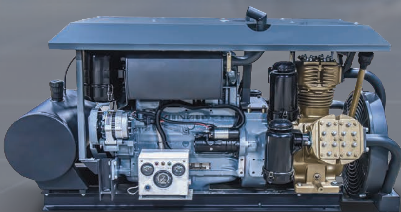
G160-3 NEW DIESEL ENGINE كمبروسر 3 راس مع ماكينة جديدة
