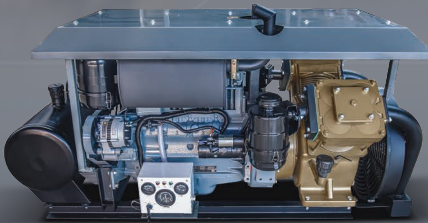
G220-2 NEW DIESEL ENGINE كمبروسر 2 راس مع ماكينة جديده
