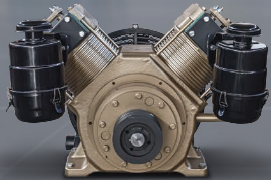
G220-2 COMPRESSOR WITH PULLEY كمبروسر 2 راس مع حزام بكرة
